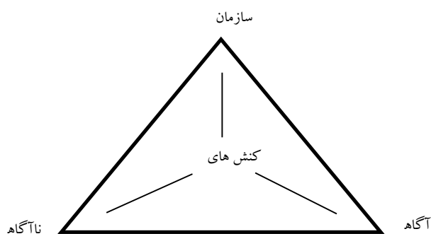
شکل ۱: سازمان کنش
