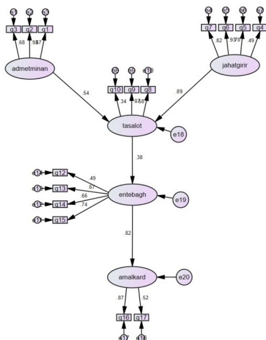
شکل ۳-مدل ساختاری برای آزمون فرضیه‌های پژوهش
